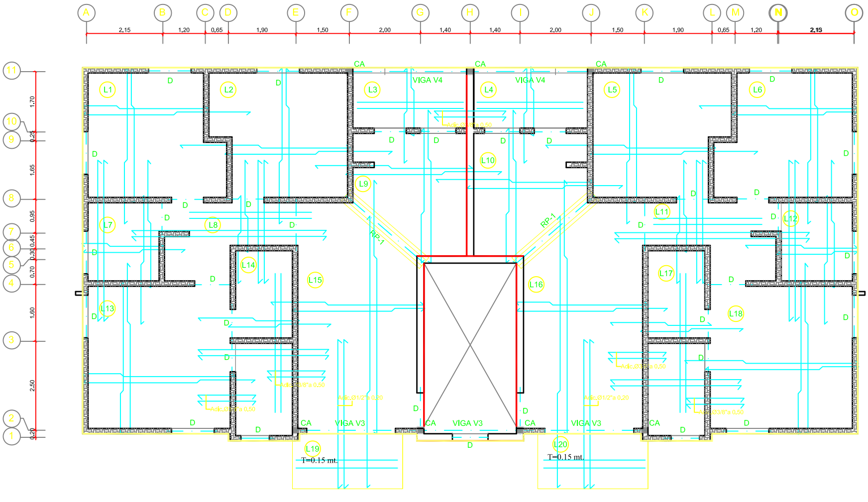
PLANTA ESTRUCTURAL DE TECHO, BLOQUE B ESCALA: 1:75
