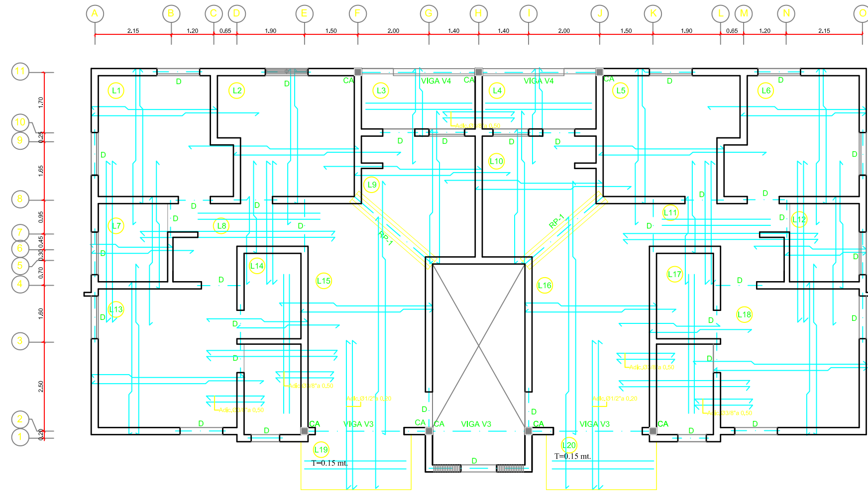
PLANTA ESTRUCTURAL 2DO. NIVEL, BLOQUE B ESCALA: 1:75
