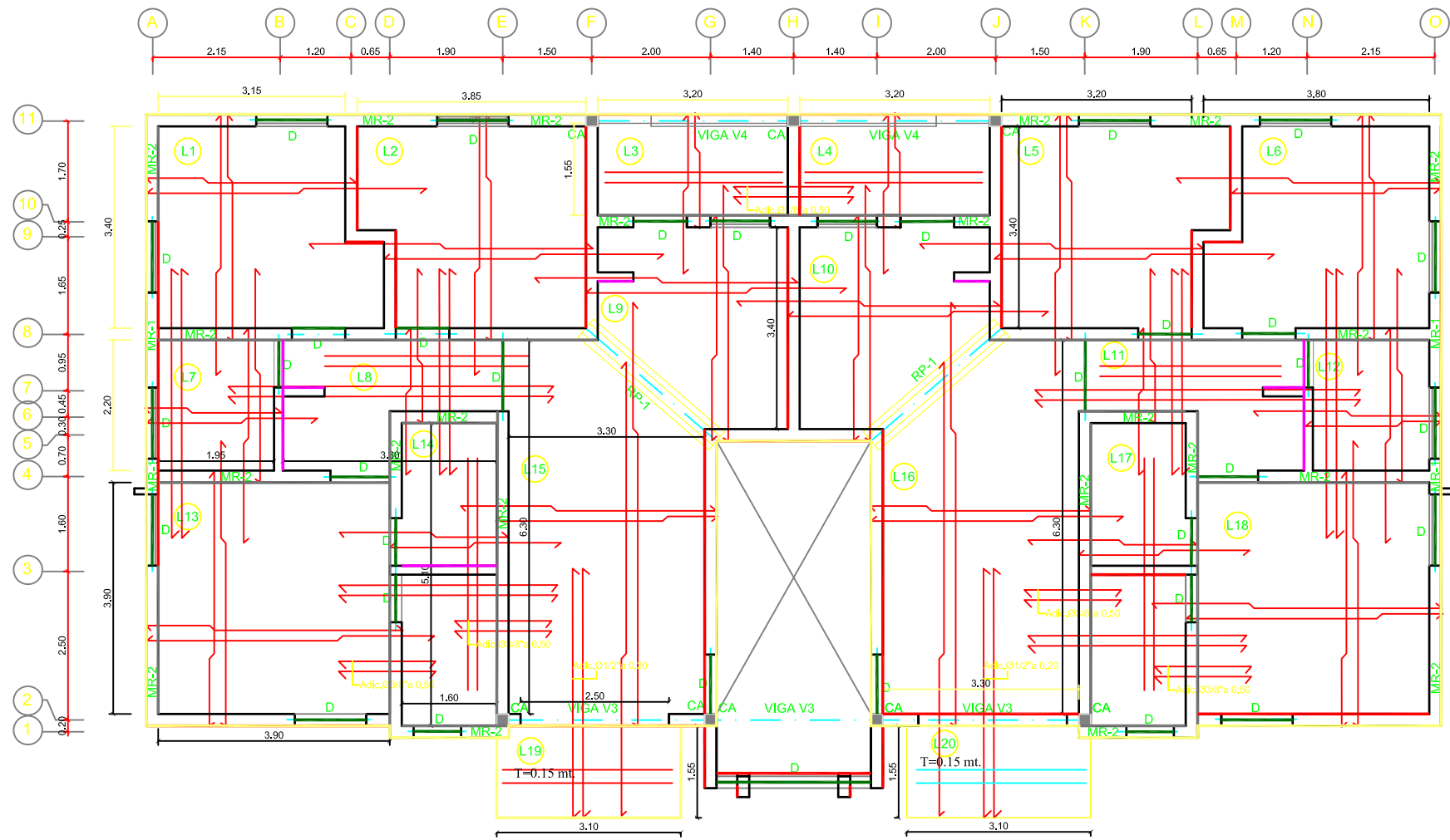
PLANTA ESTRUCTURAL 1ER. NIVEL, BLOQUE B ESCALA: 1:75
