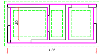
PLANTA DE CIMIENTOS GARITA ESCALA: 1:75 3 E-01
