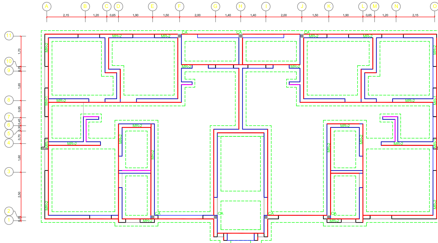
PLANTA DE CIMENTOS, BLOQUE B ESCALA: 1:75 1 E-01
