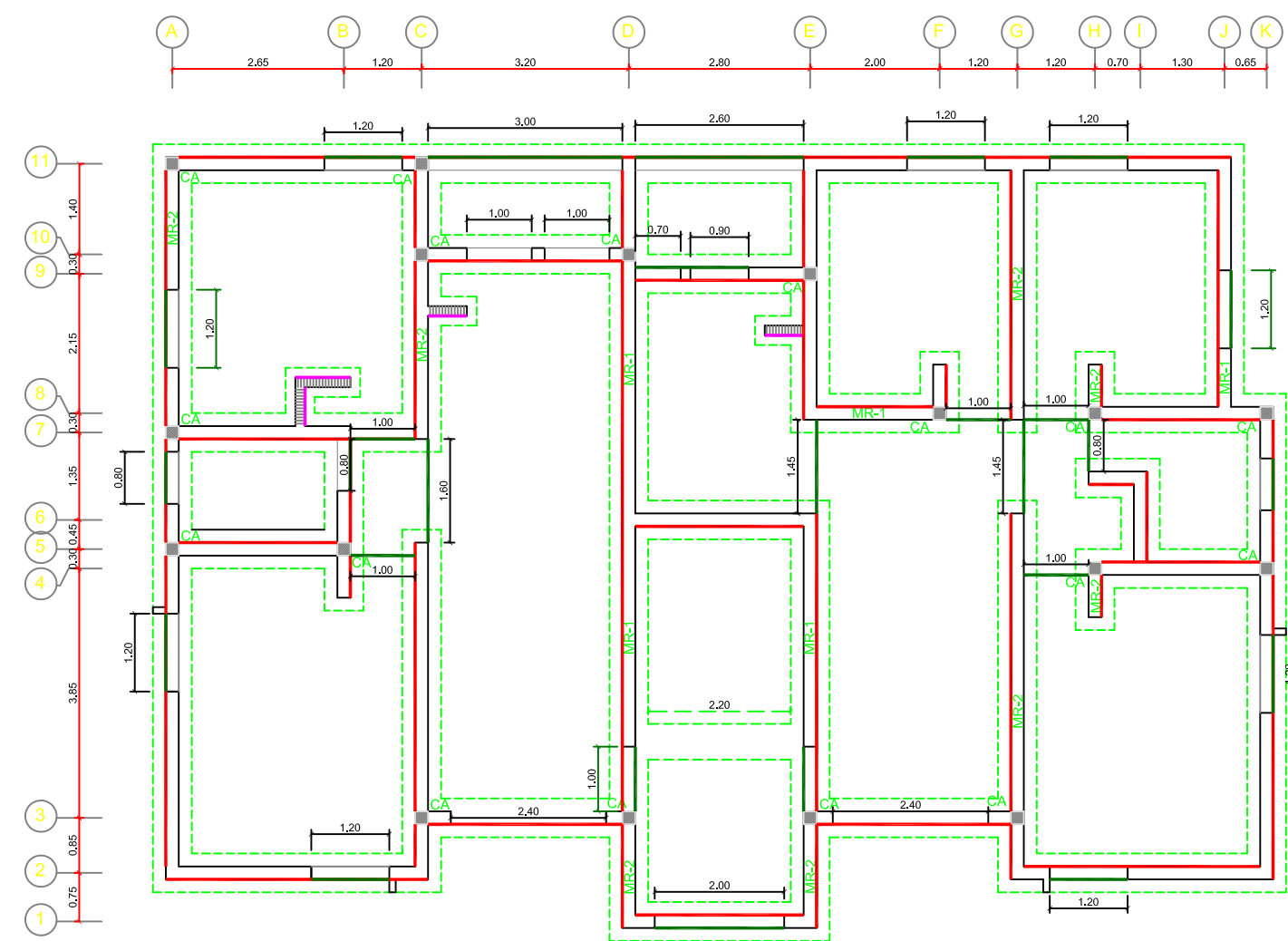
PLANTA DE CIMIENTOS, BLOQUE A
