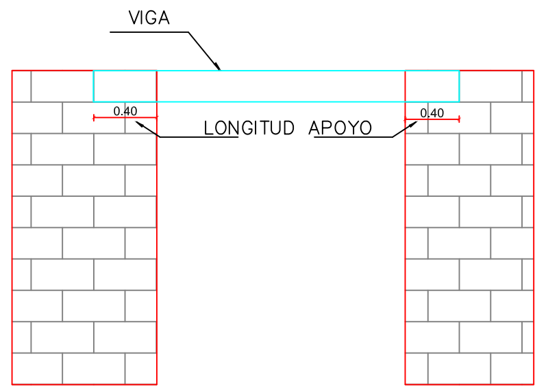
LONGITUD APOYO DE VIGA EN MUROS NO ESCALA
