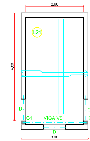
PLANTA ESTRUCTURAL TECHO ESCALERA, BLOQUE B ESCALA: 1:75
